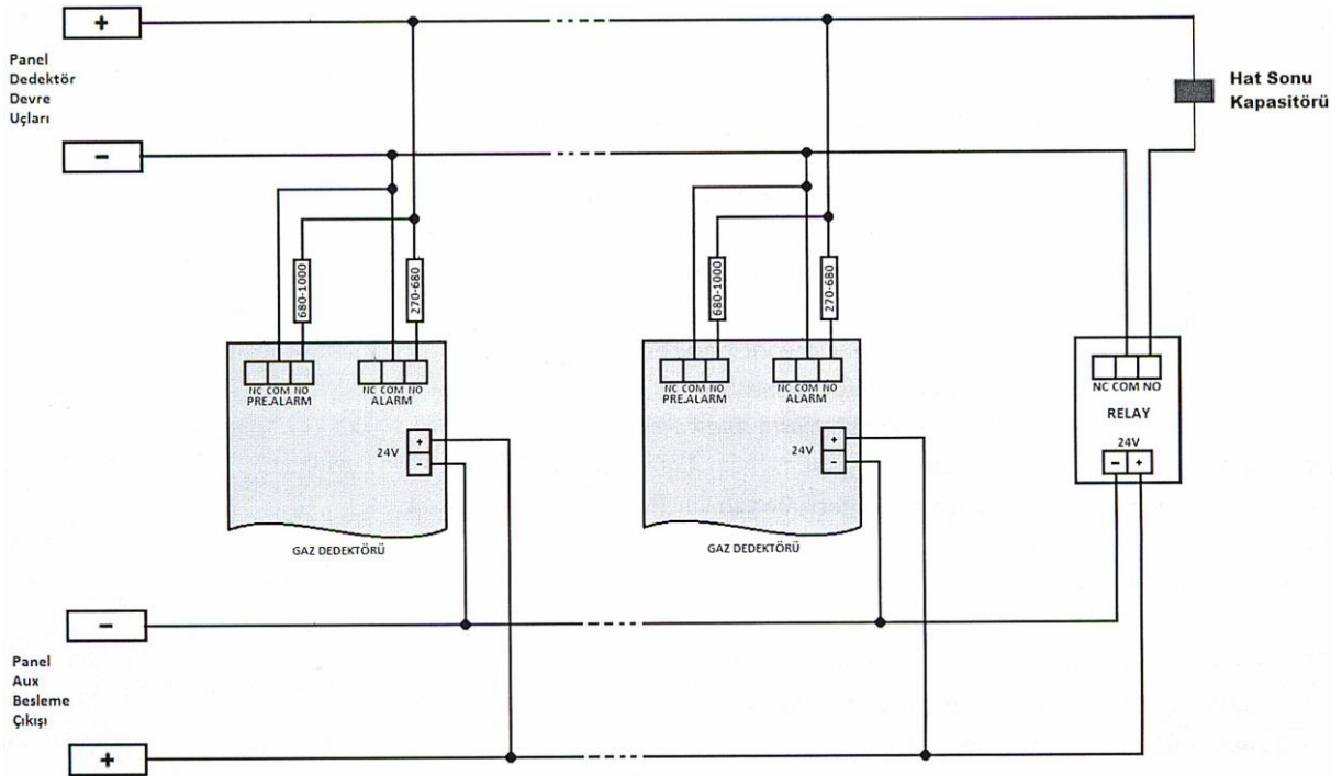
Şekil 1 – Örnek bir gaz dedektör devresi kablolama diyagramı
